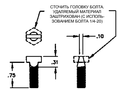
ШТИФТ СБРОСА
